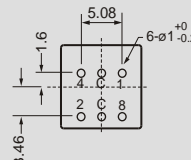
Furação do Circuito Impresso Vista por cima
